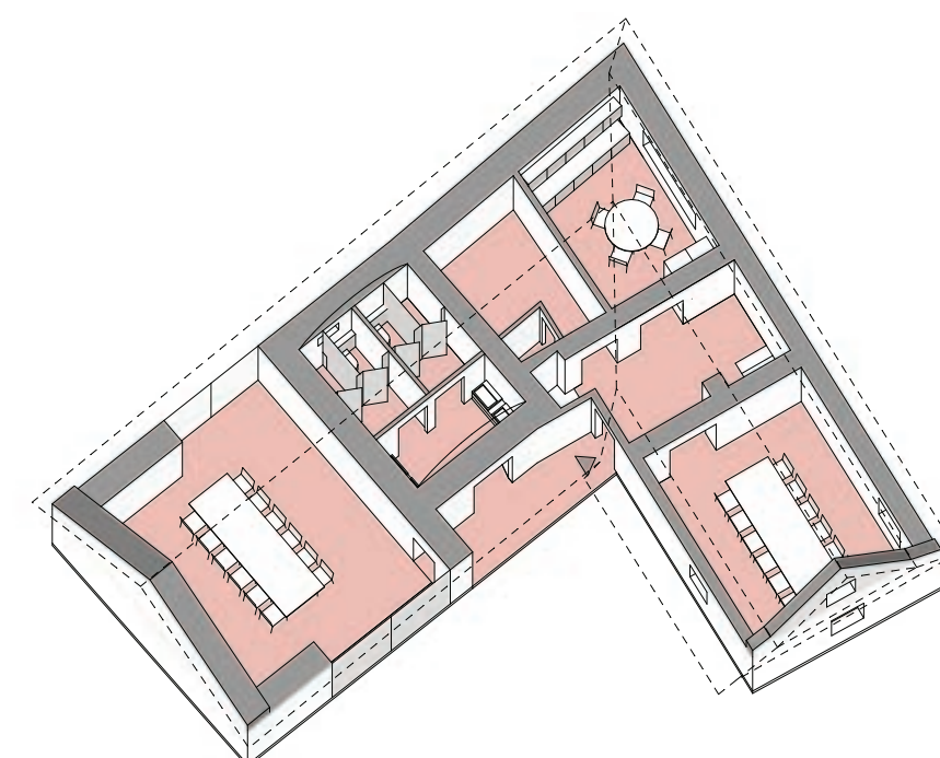
2. SPOLKOVÁ KLUBOVNA „RYBÁRNA“
